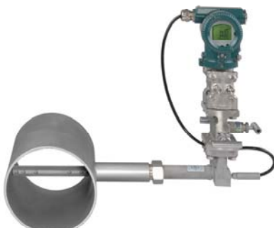
Abbildung 2: deltaflow mit Schneidringstutzen, integrierter Temperaturmessung, Dreibegeblock und multivariablen Differenzdrucktransmitter
