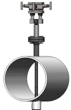
Abbildung 1 DF44 mit Flanschanschluss, Gegenlager und Dreibegeblock
