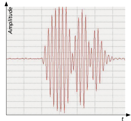
Codierte Signale: Typisches Signalkomplex mit zwei 180°-Phasenverschiebungen für zuverlässige Signalerkennung.
