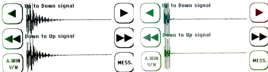
Abbildung 23: Wandler angeschlossen, kein akustischer Kontakt (ohne Magnalube)
