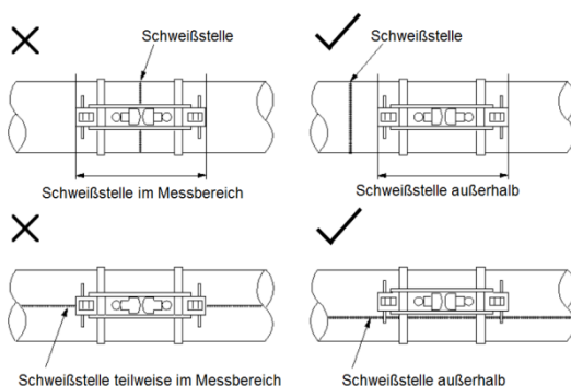
Abbildung 6: Ultraschallwandler-Montage / -Positionierung
