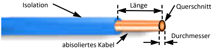
Abbildung 3: Kabelkonfektionierung
