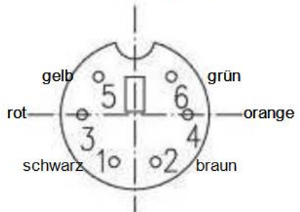
Ansicht Steckseite:
