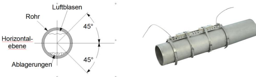
Abbildung 5: Ultraschallwandler-Montage – Positionierung (2)
