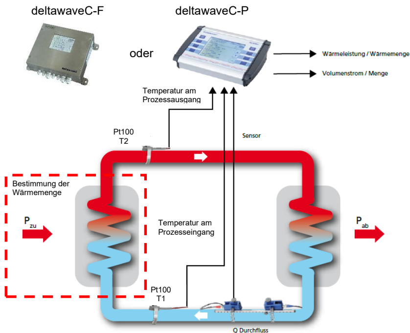
Abbildung 21: Schema Wärmemengenmessung Das deltaxwaveC-F/P zeigt Ihnen die Wärmeleistung und die akkumulierte Wärmemenge an.
