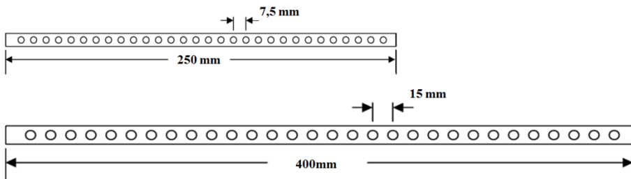
Abbildung 29: Montageschiene; oben: „kurz“, unten: „lang“
