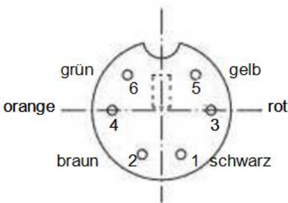
Ansicht Lötseite:
